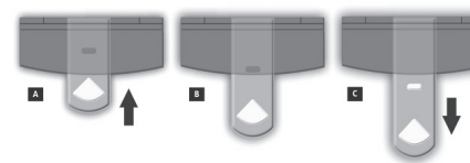
Abb. 7 Luftzufuhrregler – Typ 3
